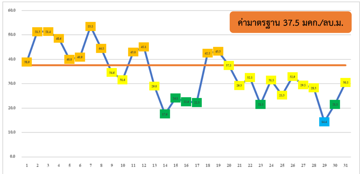
ค่าเฉลี่ย 24 ชั่วโมงของ PM_{2.5} ณ เวลา 08.00 น. ในพื้นที่จังหวัดนครปฐม เดือนธันวาคม 2567
