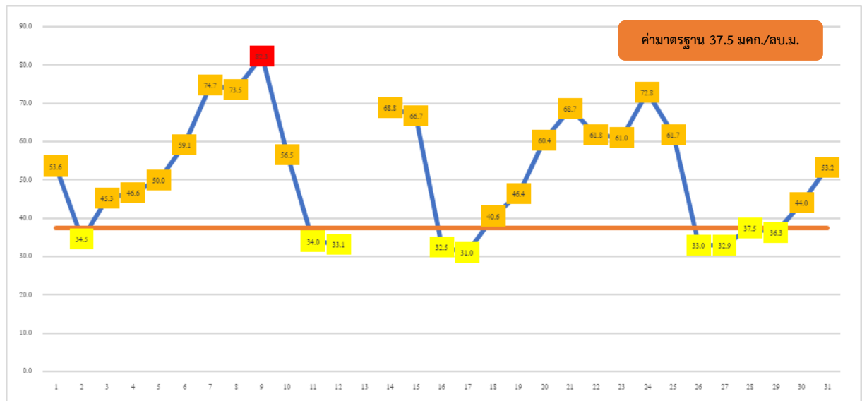
ค่าเฉลี่ย 24 ชั่วโมงของ PM_{2.5} ณ เวลา 08.00 น. ในพื้นที่จังหวัดนครปฐม เดือนมกราคม 2568
