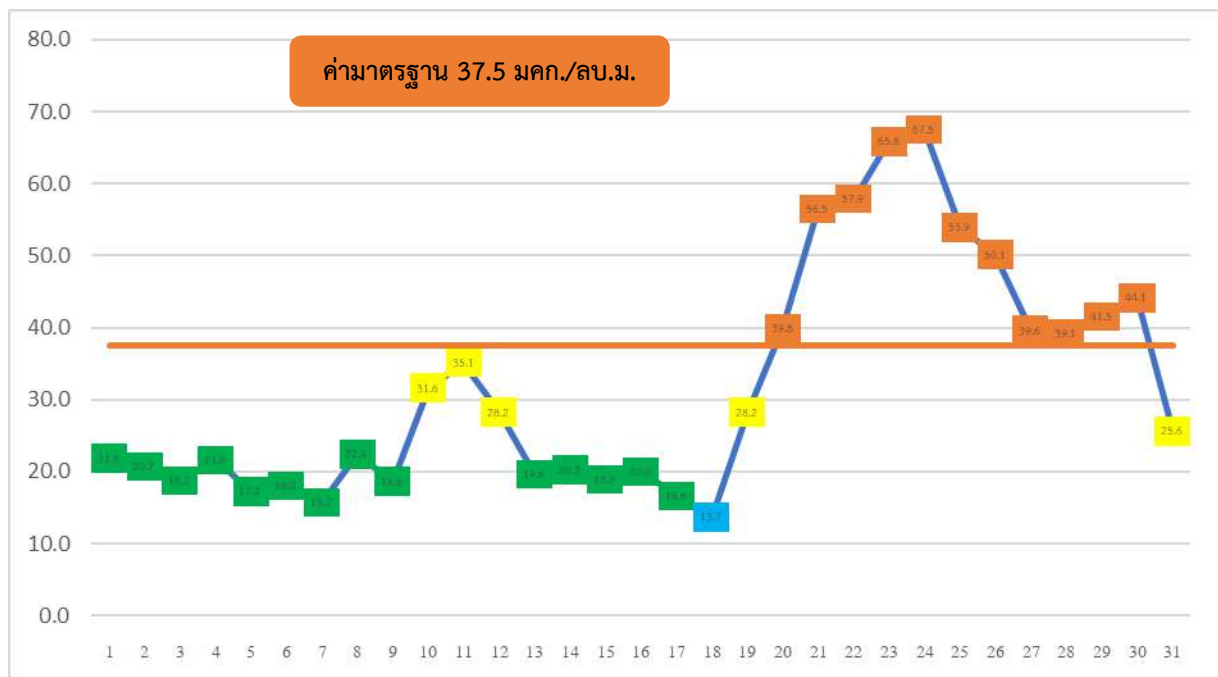
ค่าเฉลี่ย 24 ชั่วโมงของ PM_{2.5} ณ เวลา 08.00 น. ในพื้นที่จังหวัดนครปฐม เดือนมีนาคม 2568
