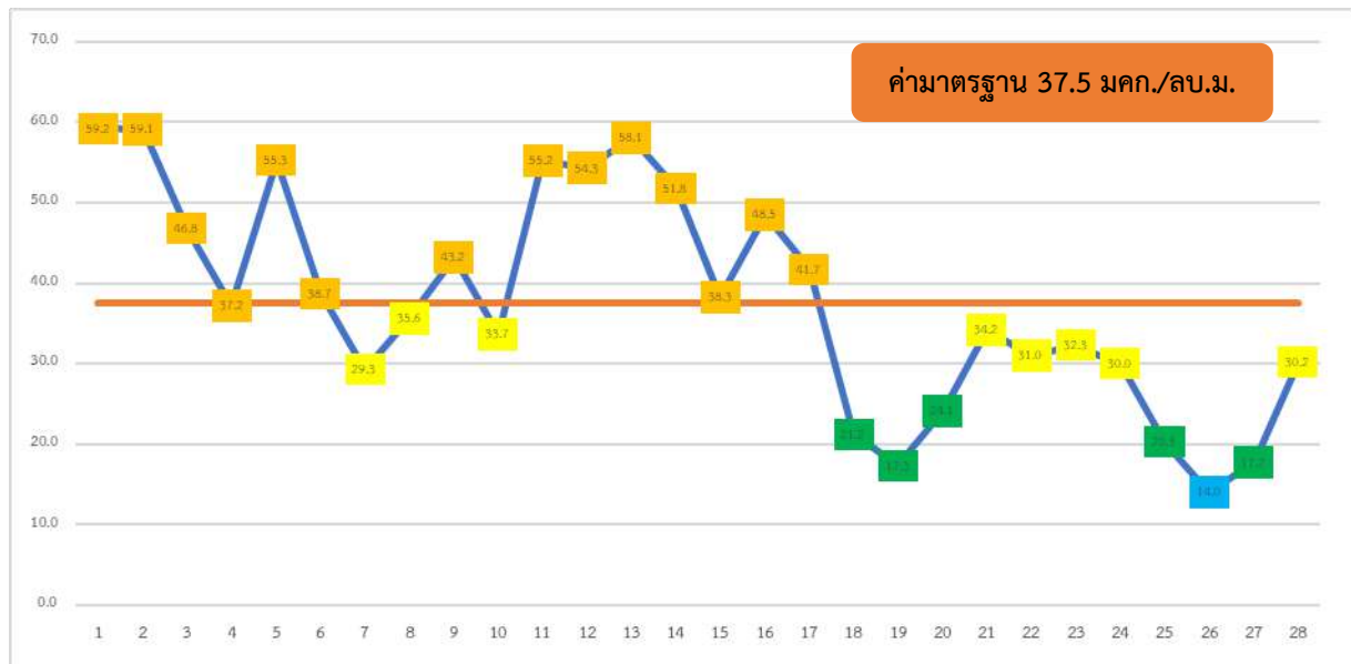
ค่าเฉลี่ย 24 ชั่วโมงของ PM_{2.5} ณ เวลา 08.00 น. ในพื้นที่จังหวัดนครปฐม เดือนมีนาคม 2568
